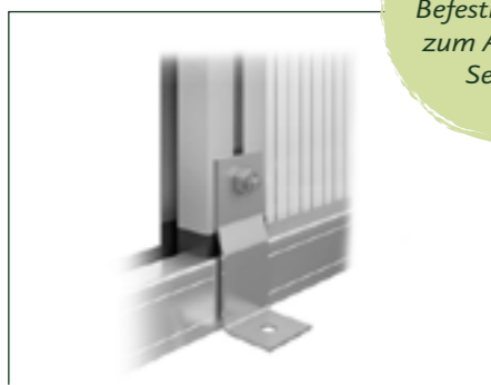
Befestigungs-Set zum Aufdübeln
